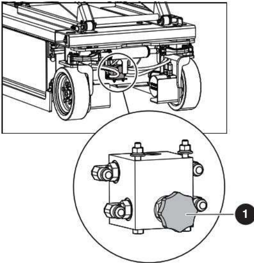
Figura 07 Válvula de livre rodagem na parte dianteira da base (SJ3215 e SJ3219)
