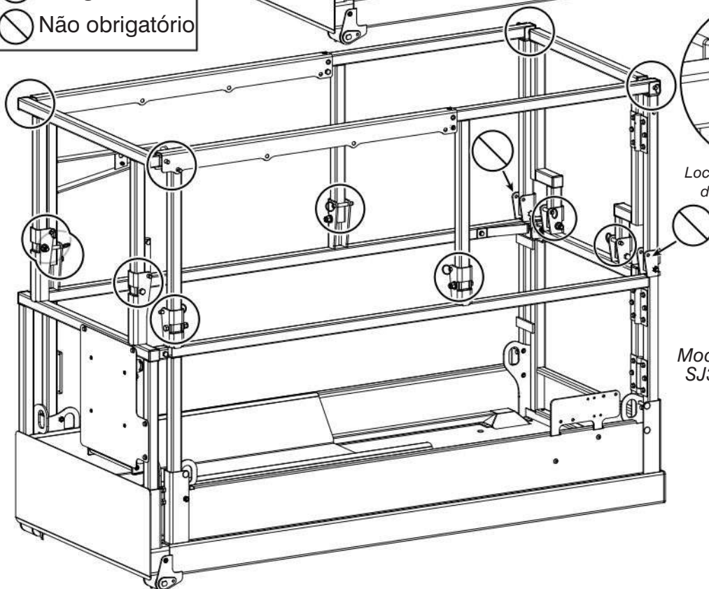
Figura 15 Localização do pino de travamento do trilho de segurança - SJ3215, SJ3219, SJ3220, SJ3226
