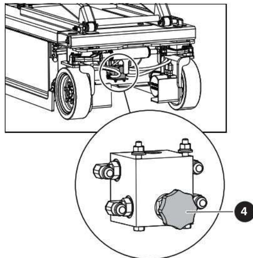
Figura 04 Válvula de livre rodagem (SJ3215 e SJ3219)
